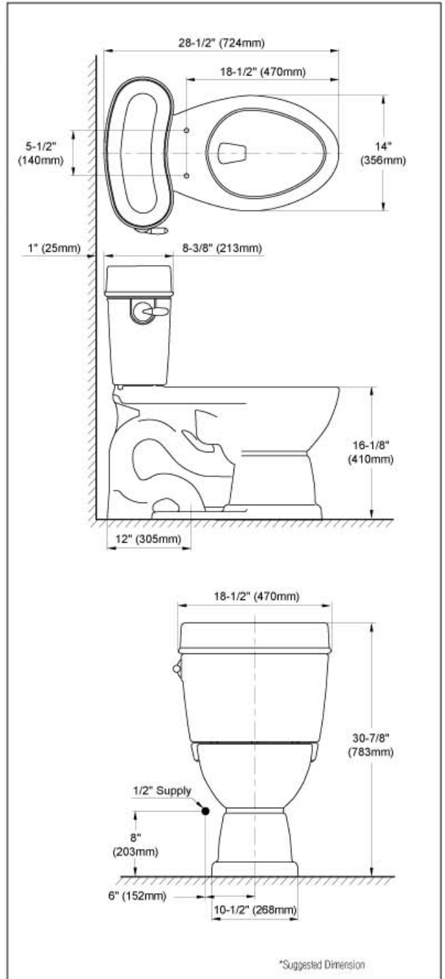
MS756204SF - Mercer™ Toilet
